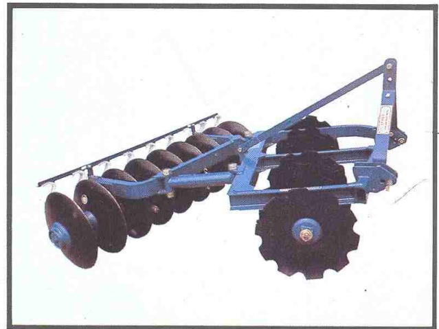
พรวน 18 จาน HR 30-18 ● HR 30-18B
