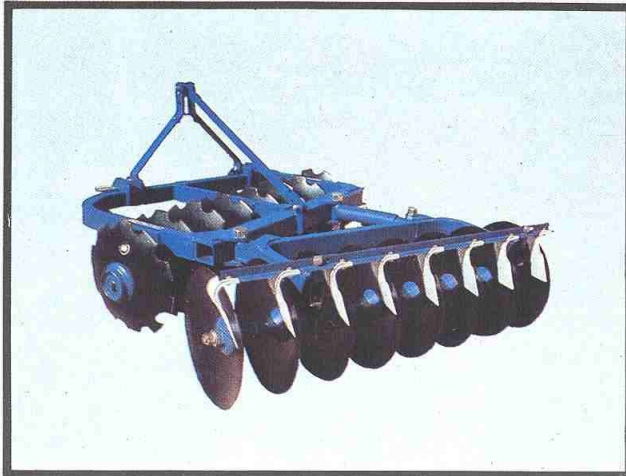
พรวน 16 จาน HR 29-16 ● HR 29-16 B
